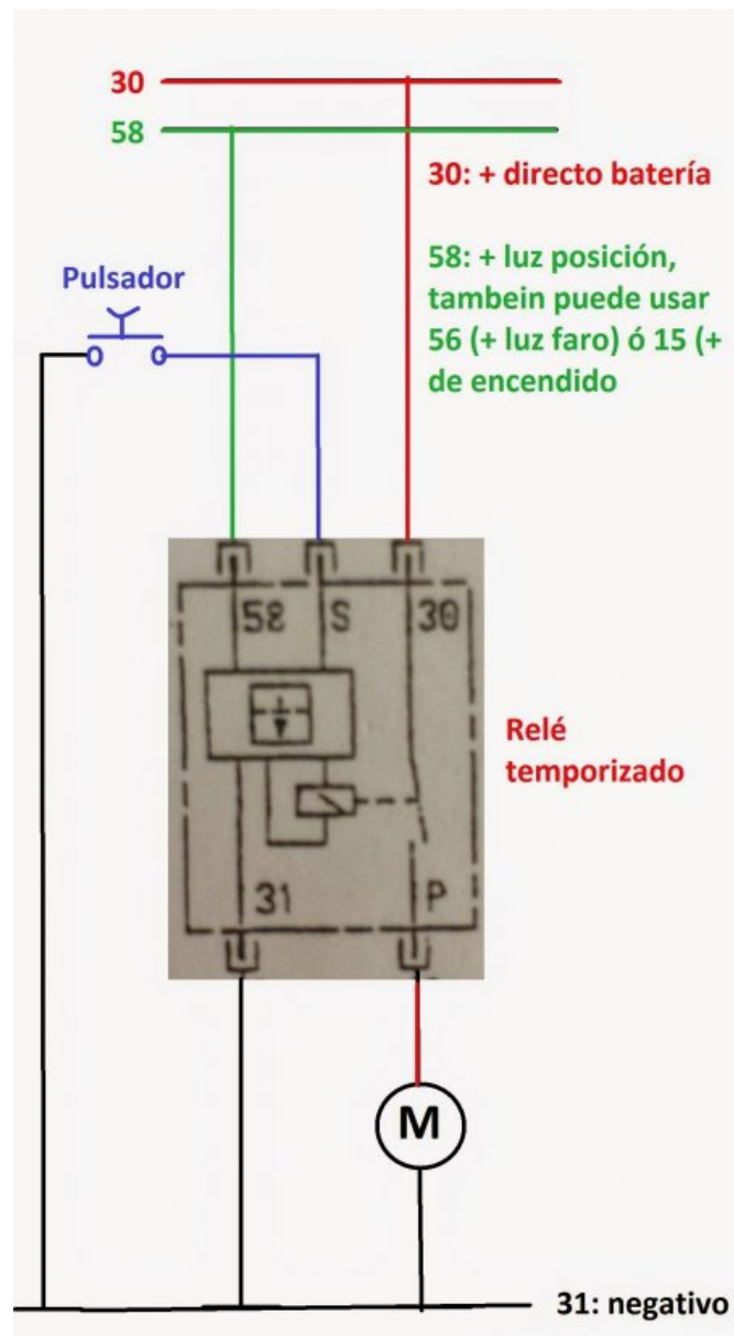
Circuito bomba limpiaparabrisas
