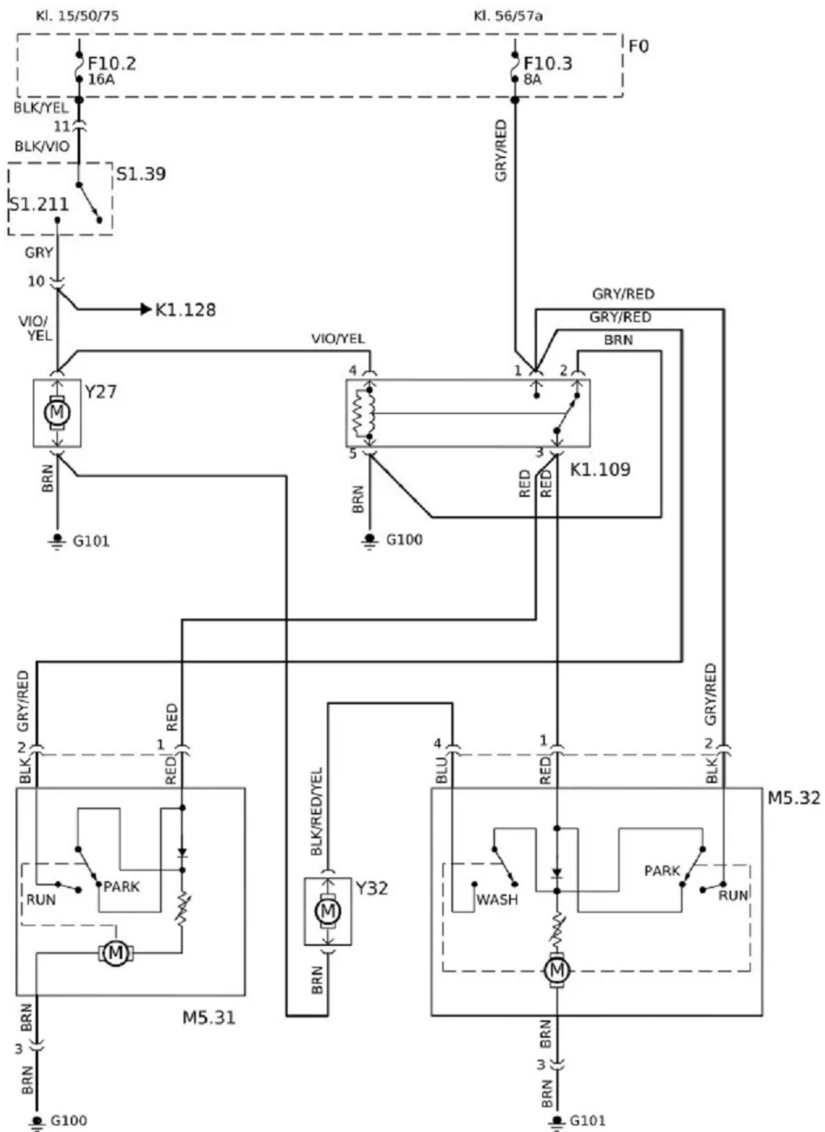
Circuito limpia y lavaparabrisas real
