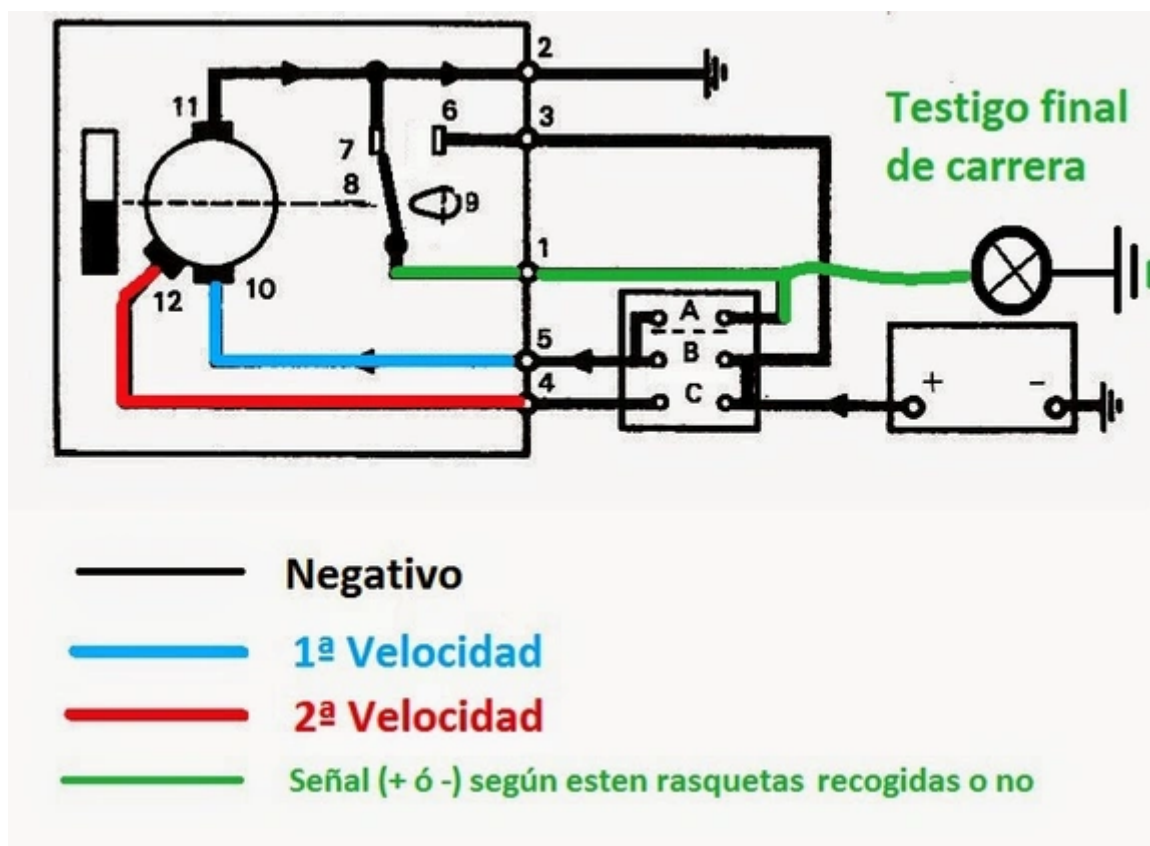
Esquema eléctrico del motor del limpiaparabrisas - Sistemas Eléctricos del Automóvil
