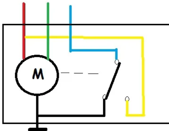
Esquema de conexión del motor del limpiaparabrisas con tres cables - Sistemas Eléctricos del Automóvil
