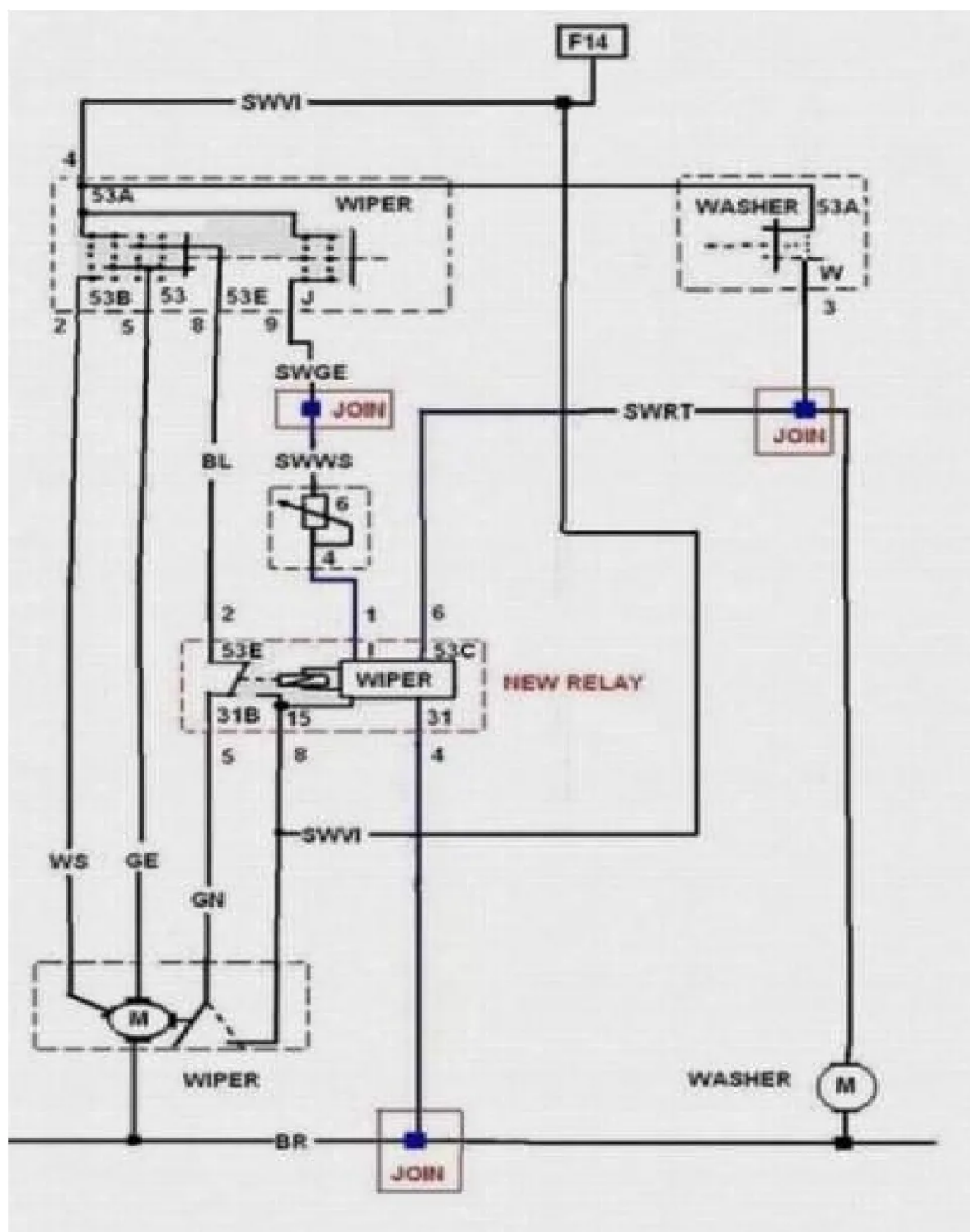
Circuito limpiaparabrisas con cadenciación programable
