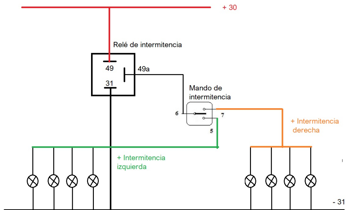
Circuito de intermitencias del automóvil - Sistemas Eléctricos del Automóvil
