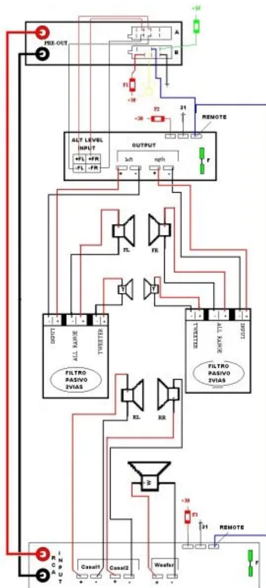
Diagramas eléctricos de sonido en el automóvil con altavoces y tweeters (con filtros) delanteros amplificados y altavoces y woofer traseros amplificados
