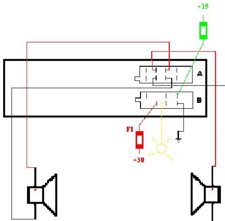
Circuito con dos altavoces delanteros y tweeters en el salpicadero (con filtro incorporado)
