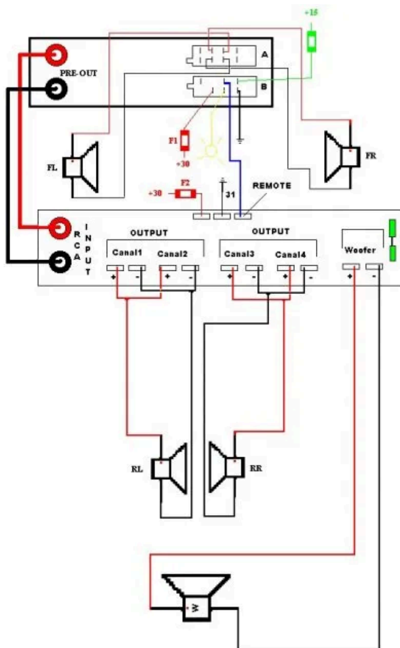
Instalación con dos altavoces delanteros y dos traseros con woofer amplificados (típica juvenil)
