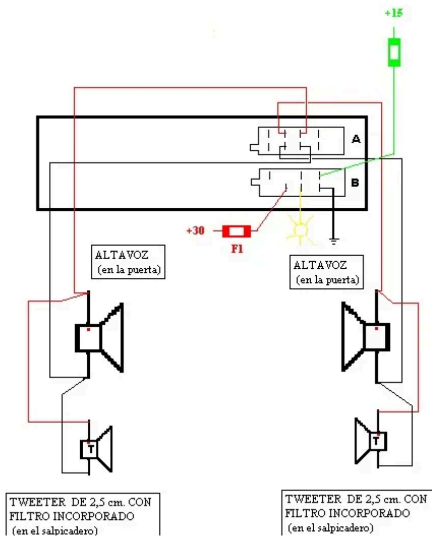
Circuito con dos altavoces delanteros y tweeters en el salpicadero (con filtro incorporado)
