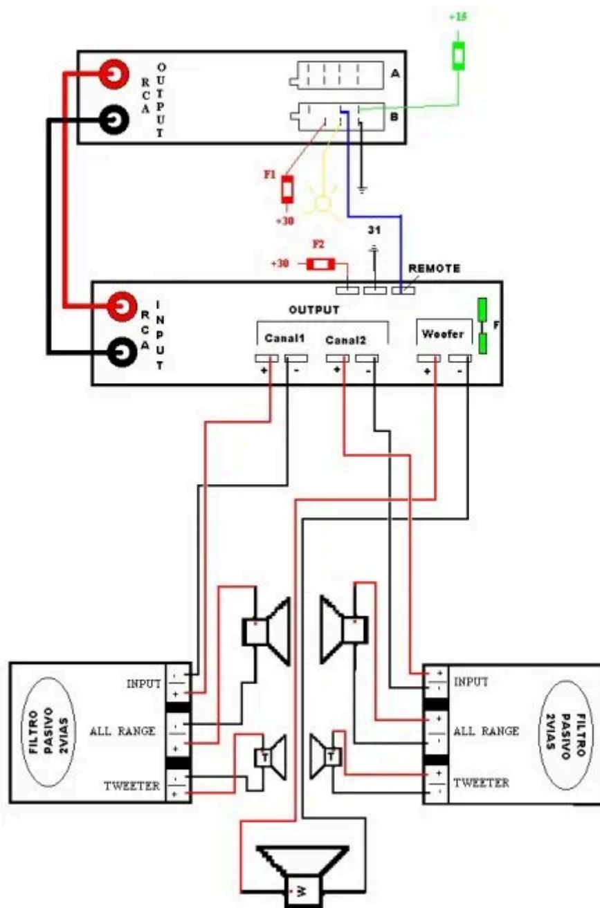
Diagramas eléctricos de sonido en el automóvil Instalación de altavoces delanteros con etapa 3-2 filtros de 2 vías woofer y tweeters
