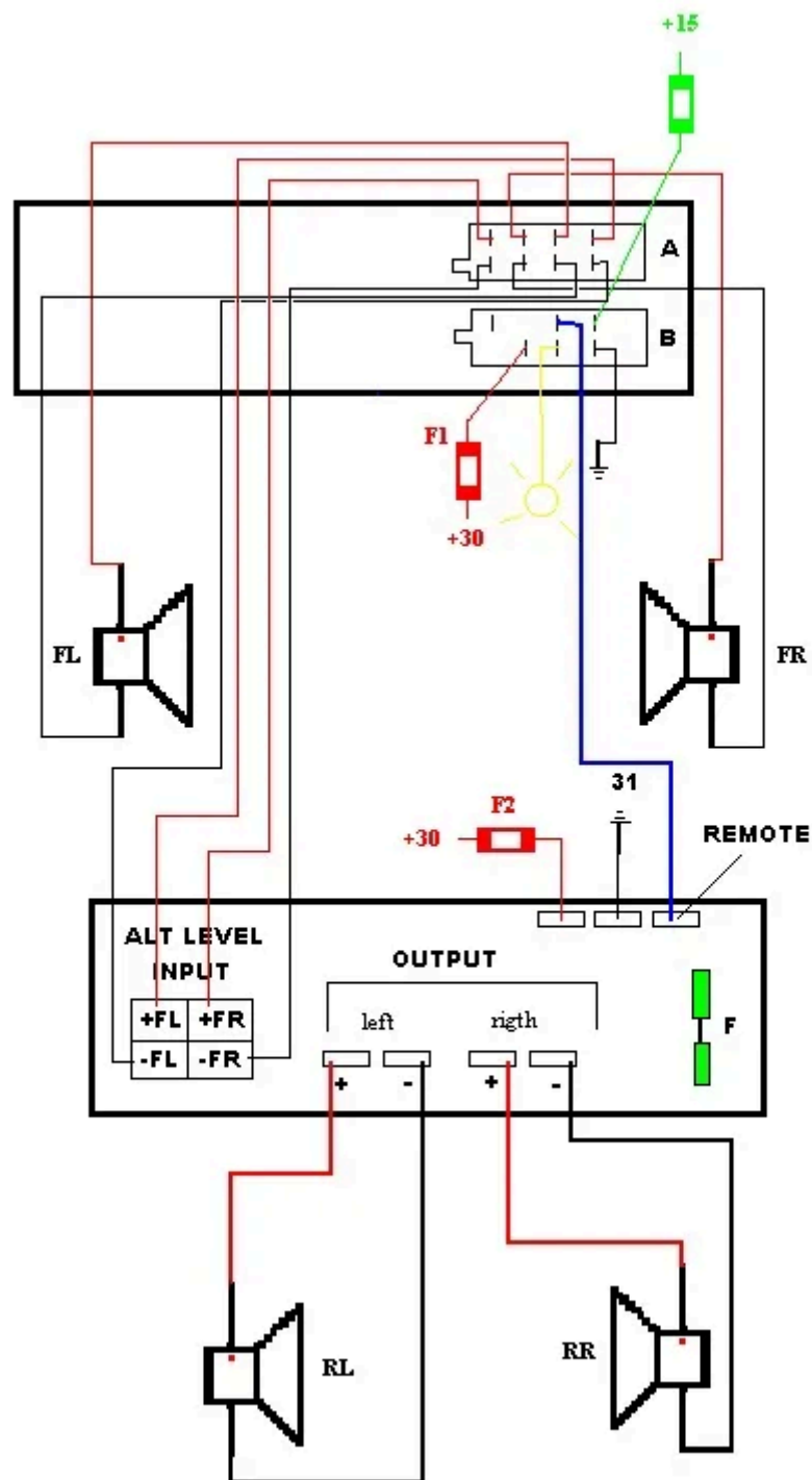
Diagramas eléctricos de sonido en el automóvil con dos altavoces y tweeters (con filtros) delanteros amplificados y altavoces y woofer traseros amplificados
