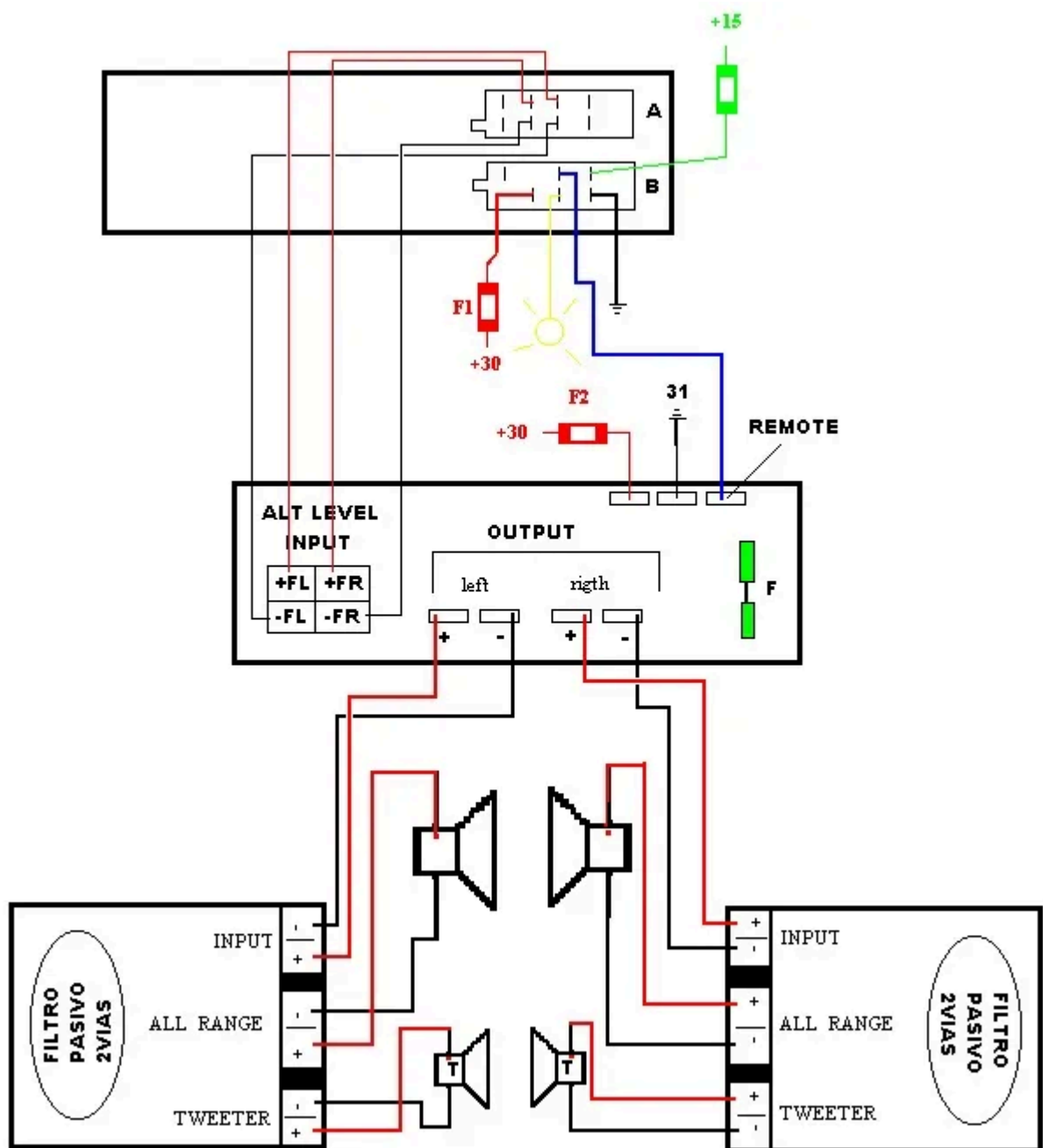
Instalación de altavoces delanteros con etapa de potencia, tweeters y filtros pasivos de dos vías (kit)
